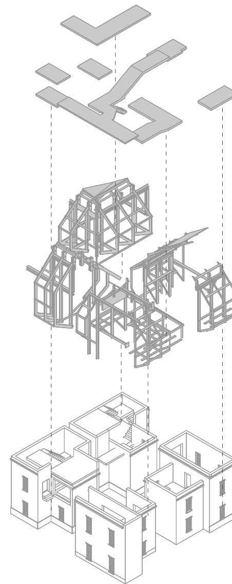
Axonométrica desglosada. TFC B – UB.
